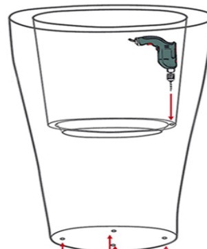
Bohrlöcher für unbeleuchtete Pflanzgefäße bei Outdoor-Einsatz Drill holes for unlit planters for outdoor use Trous de forage pour les jardinières non éclairées en cas d'utilisation en extérieur Fori per fioriere non illuminate da esterno Taladros para jardineras sin iluminación para exteriores Wiercenie otworów pod niepodświetlane donice do użytku zewnętrznego
