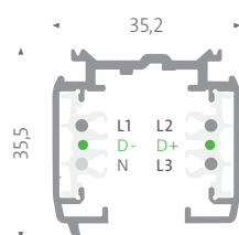
PRO-06 3-PHASEN DALI AUFBAUSCHIENE
