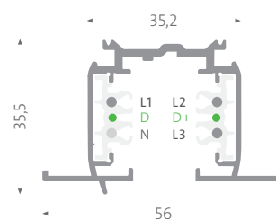
PRO-R6 3-PHASEN DALI EINBAUSCHIENE
