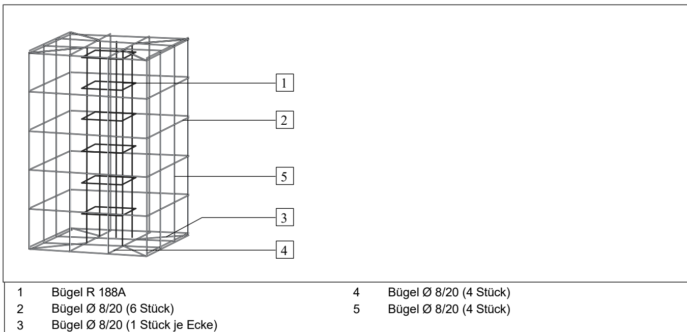
Abb. 2: Bewehrung binden
