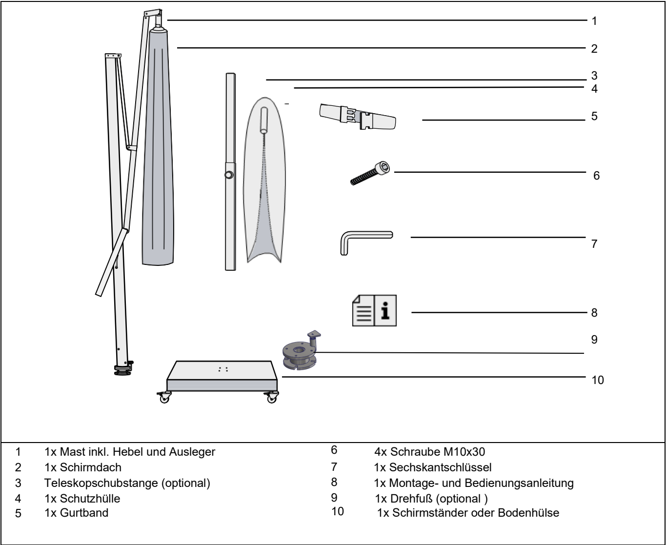
Abb. 1: Lieferumfang
