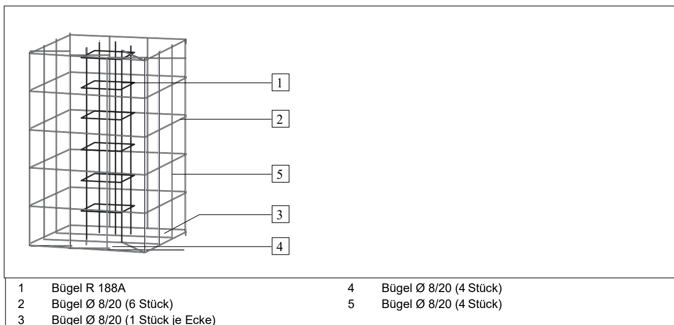
Abb. 4: Bewehrung binden
