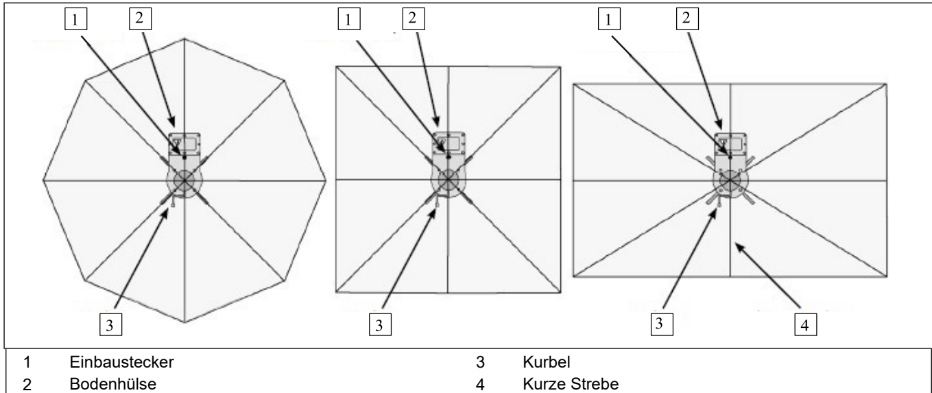
Abb. 5: Bodenhülse für Ausrichtung beachten
