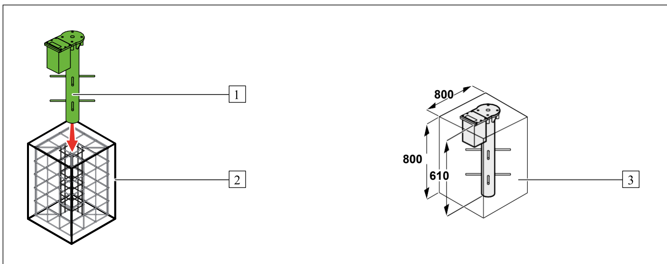
Abb. 6: Vorgehen Bodenhülse einbetonieren
