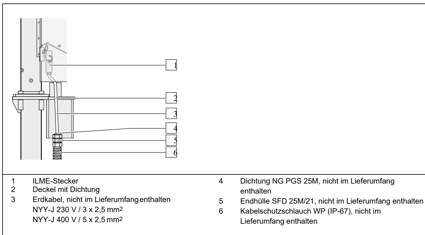
Abb. 7: Erdkabel anschließen
